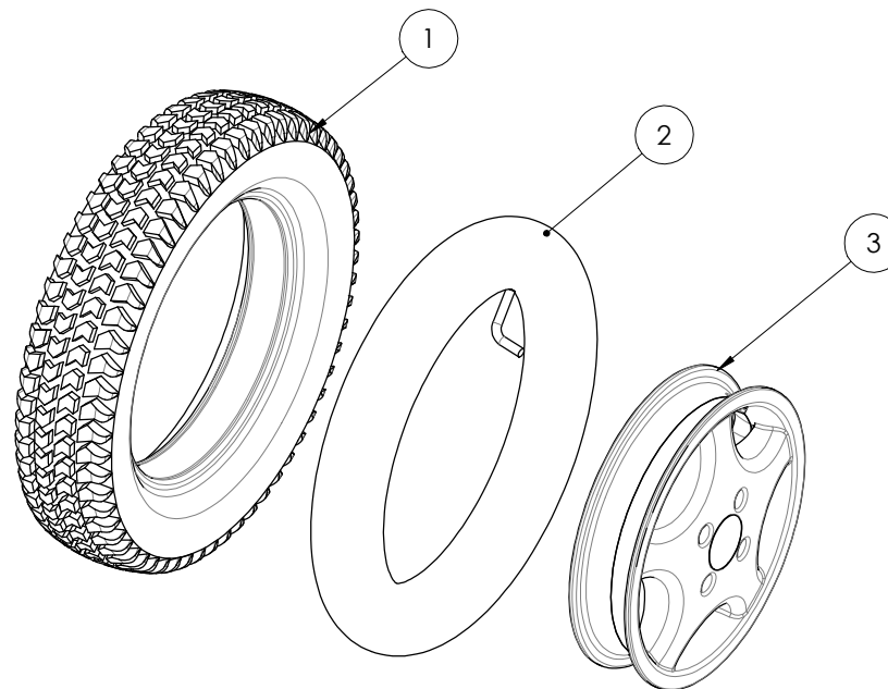
7350006081613 - Drivhjul 13" luft grå Modell H
