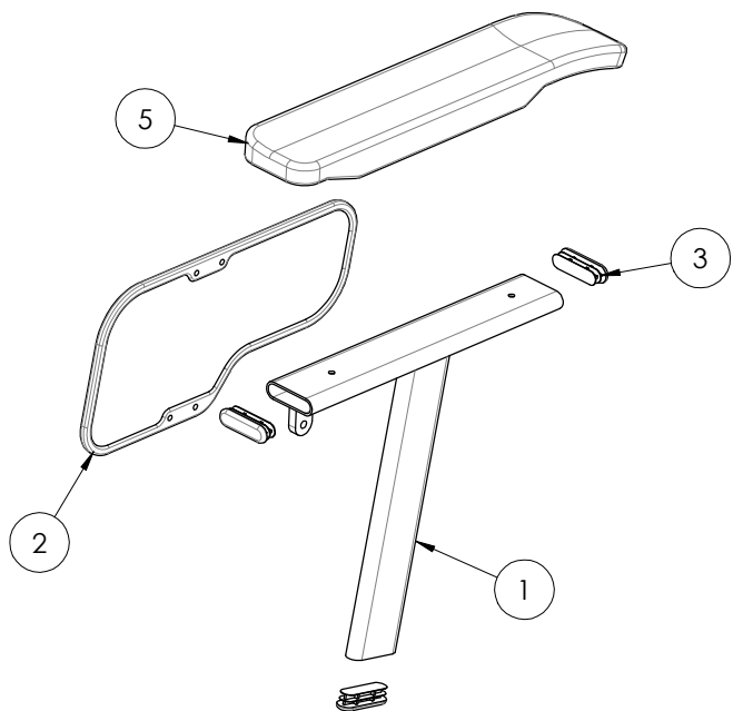
7350006081996 - Armstöd komplett HÖ Modell H (BILD OVAN):
